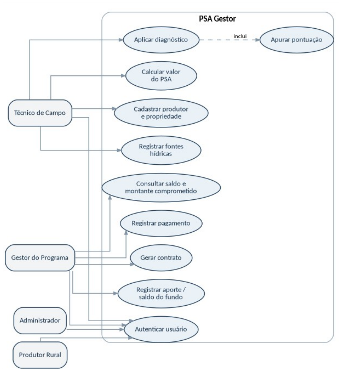
Figura 2 — Visão geral dos casos de uso detalhados.
